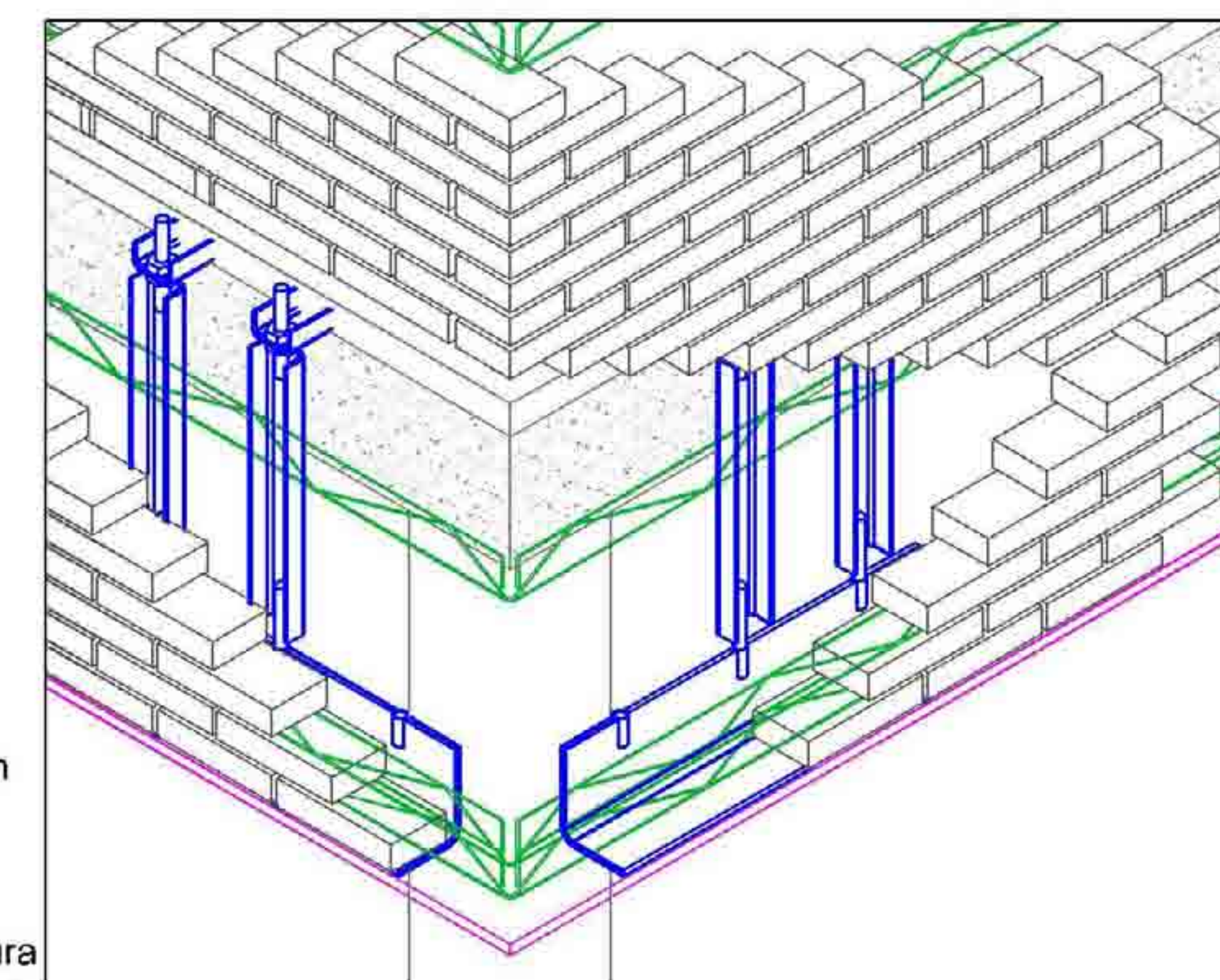
APOYO ALLWALL PI DE CUELQUE Y ESQUINA
