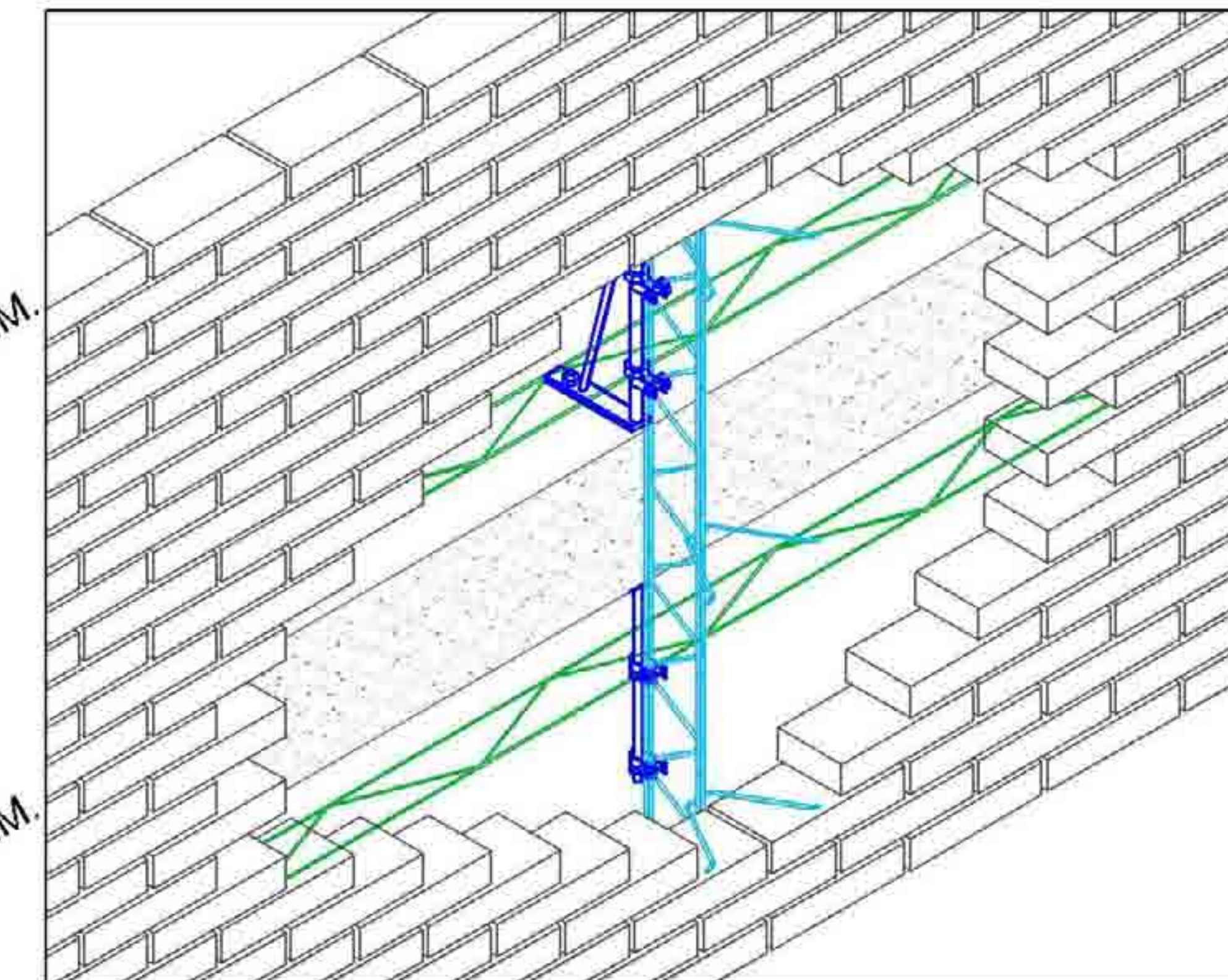
PETO DE CUBIERTA CON COSTILLA ALLWALL
