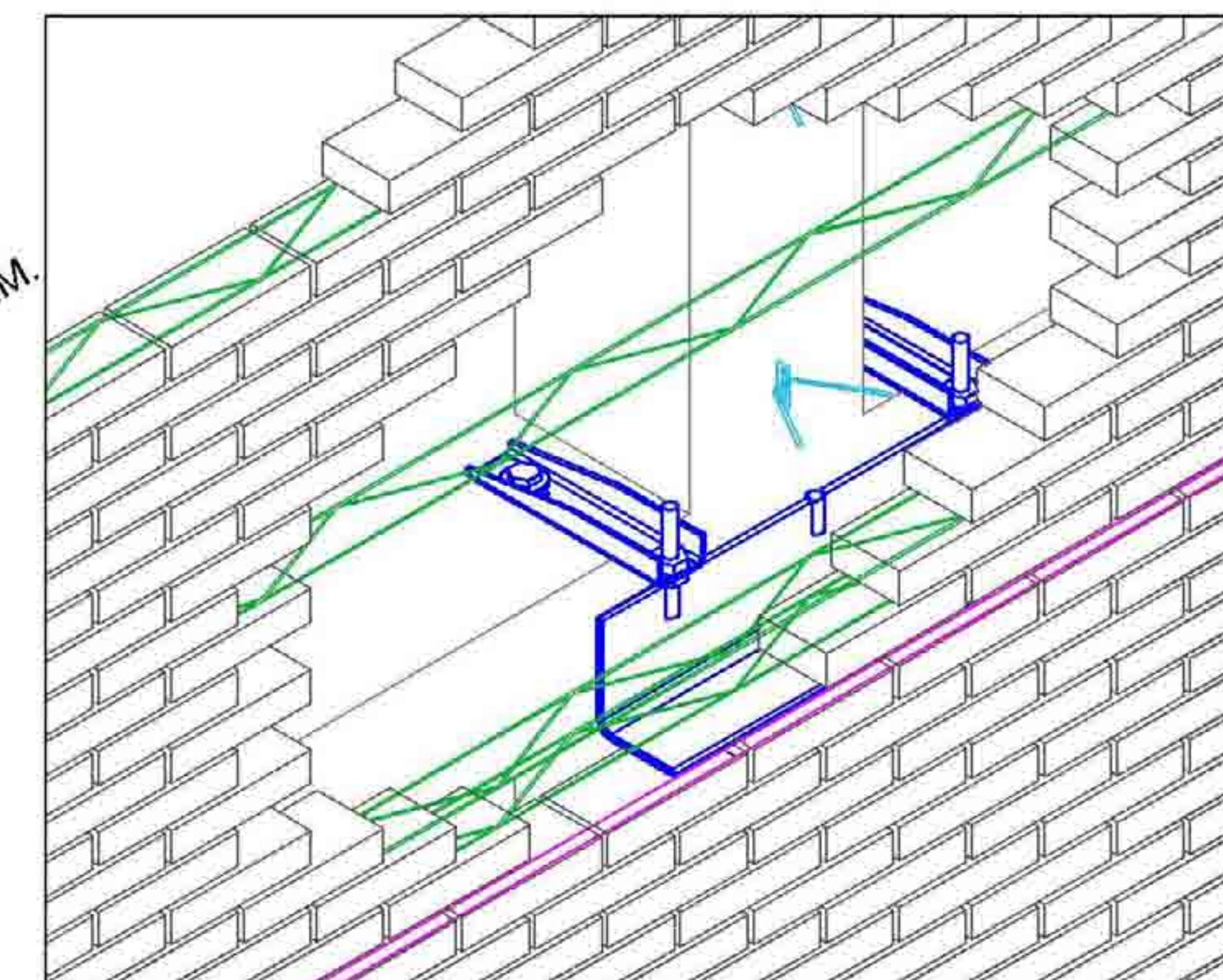
APOYO ALLWALL PI JUNTO AL PILAR
